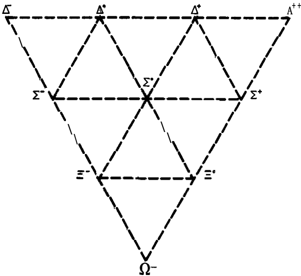
the baryon decuplet
