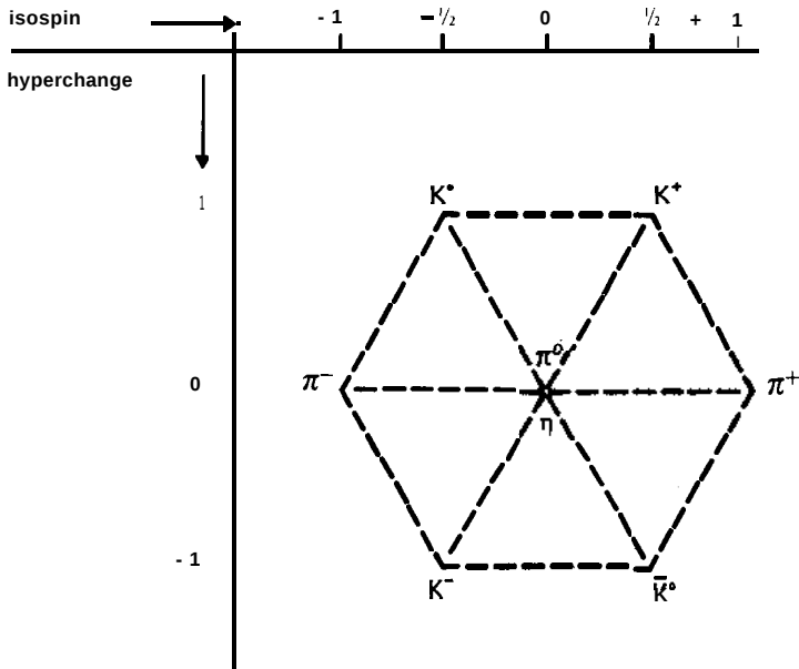
the meson octet
