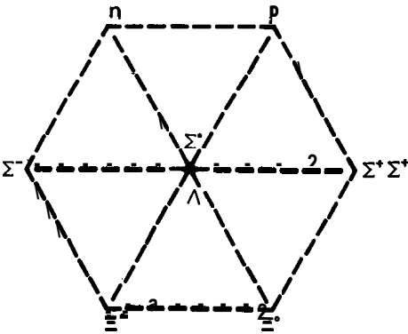
the baryon octet
